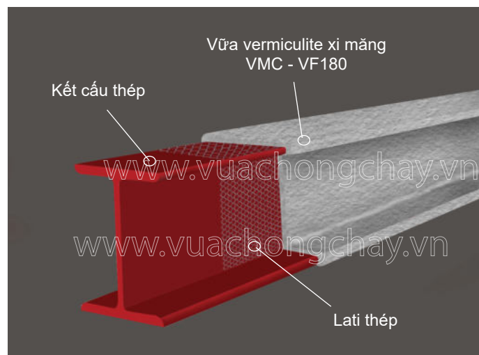
Phun bảo vệ đặc cho dầm
